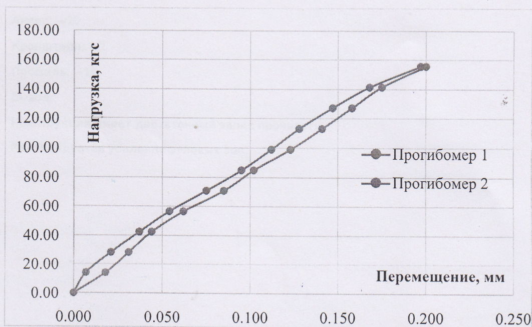
Рисунок 6. Диаграмма зависимости между приложенной вертикальной нагрузкой и вертикальным перемещением
