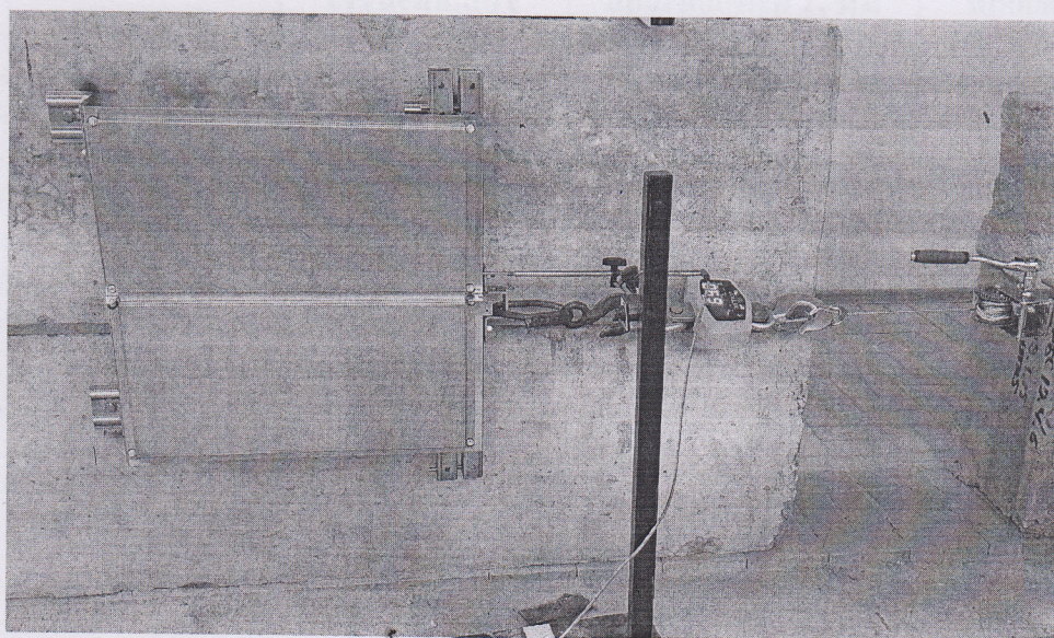
Рисунок 3. Общий вид металлического изделия замаркированного «образец №1 – навесной фасад, КУ 150x80» при сдвигающей нагрузке
